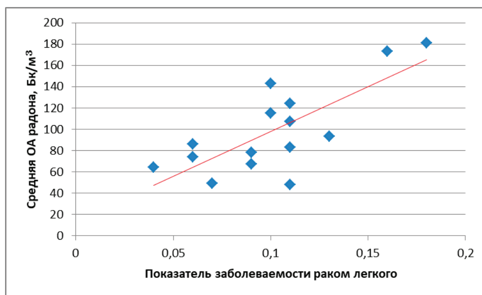
Рис. 1. Зависимость между средними значениями объемной активности (ОА) радона и показателем количества онкологических больных раком легких
